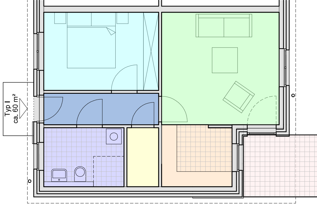
Grundrissaufteilung Typ I
